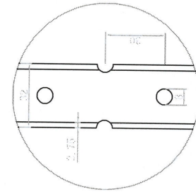
真空管详图B (mm)
